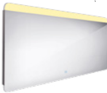
LED zrcadlo 1400 x 700 S dotykovým senzorem. Příkon 21W. Možnost nastavení teploty svítivosti od 2700K - 6000K. Rám hliníkový.
