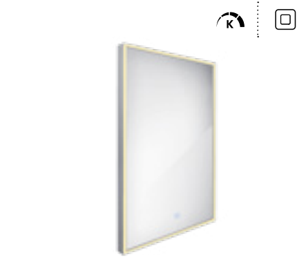
LED zrcadlo 500 x 700 S dotykovým senzorem. Možnost nastavení teploty svítivosti od 2700K - 6000K. Příkon 35W. Rám hliníkový.
